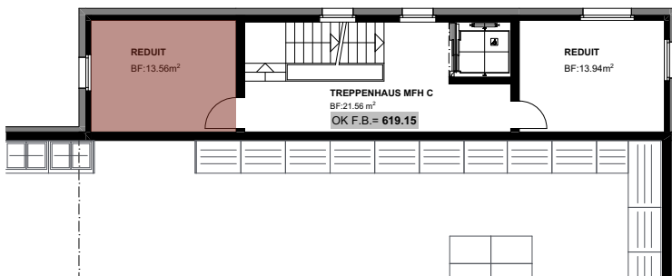
Ausschnitt ZG 1:200
