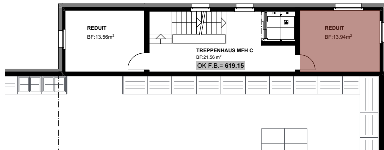
Ausschnitt ZG 1:200
