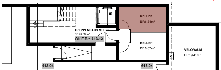
Ausschnitt UG 1:200
