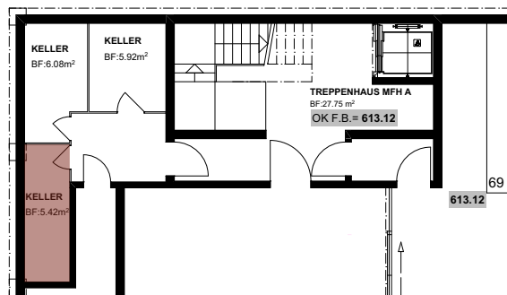
Ausschnitt UG 1:200
