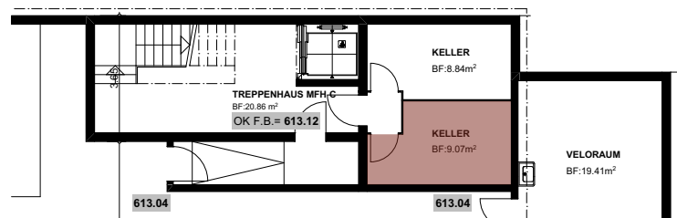
Ausschnitt UG 1:200
